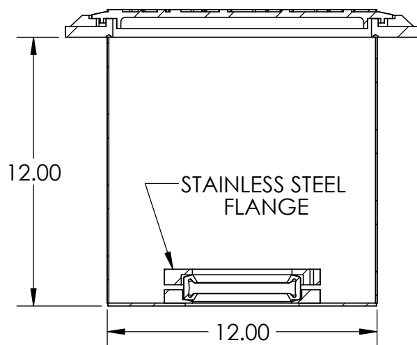
SECTION D-D
